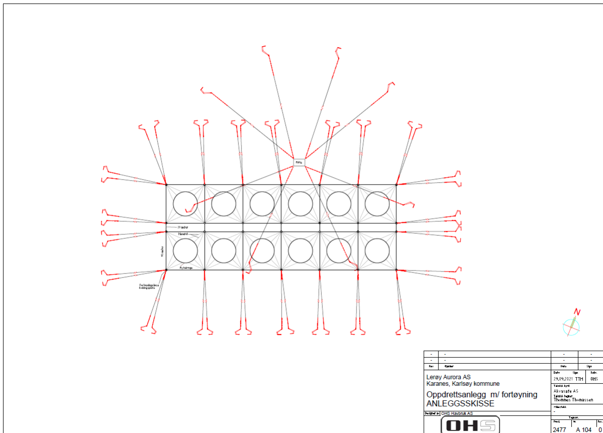
Figur 4 Karanes -A104 Anleggsskisse
