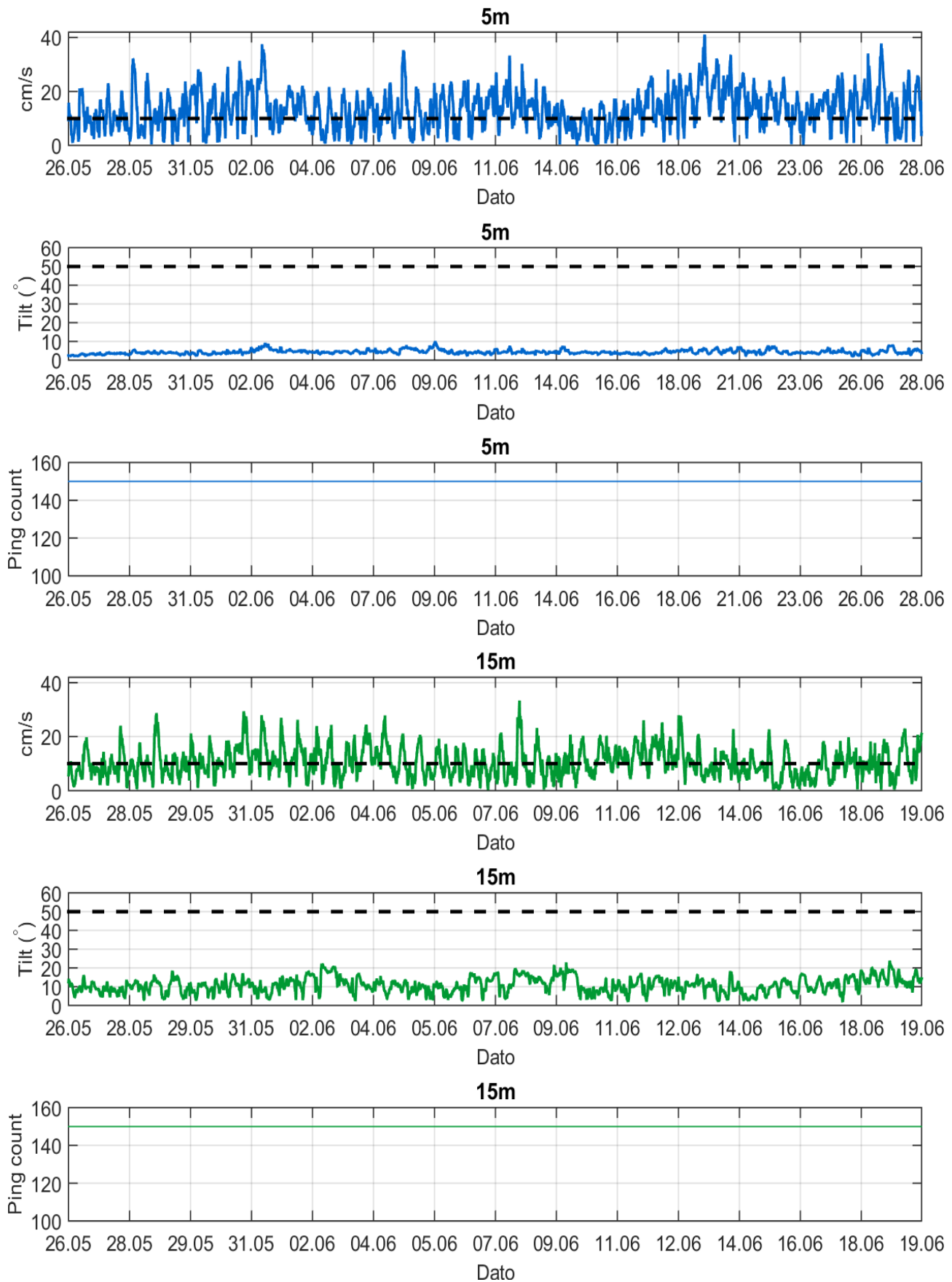
Figur 8.2.1. Tidsdiagram – kvalitetssikring av strømshastighet med instrument tilt og ping count.
