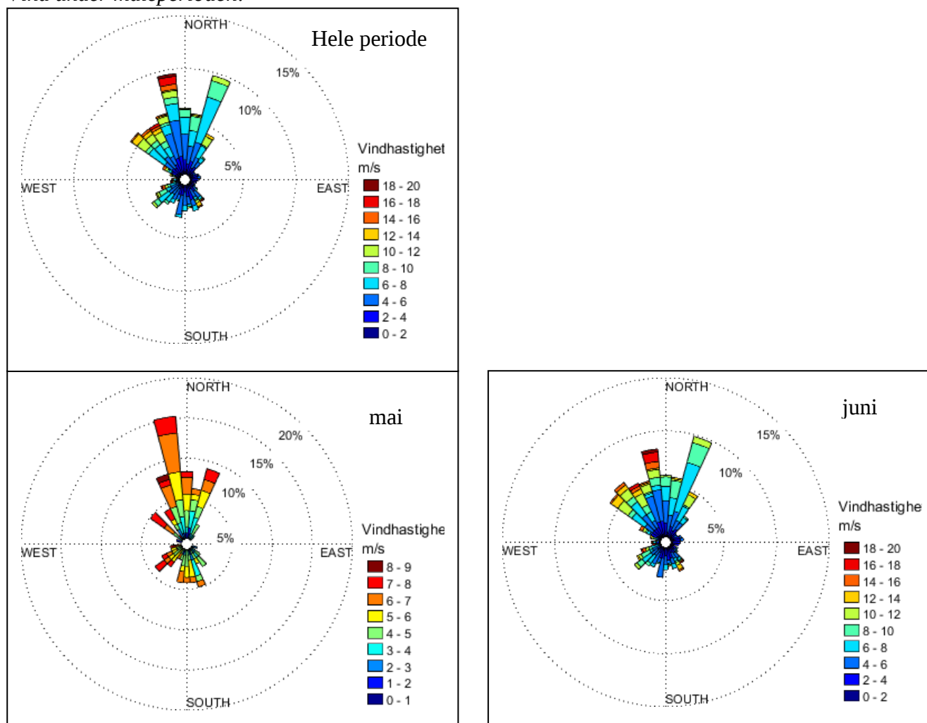
Figur 11.1. Vindrose under måleperioden fra værstasjon, Fakken.
