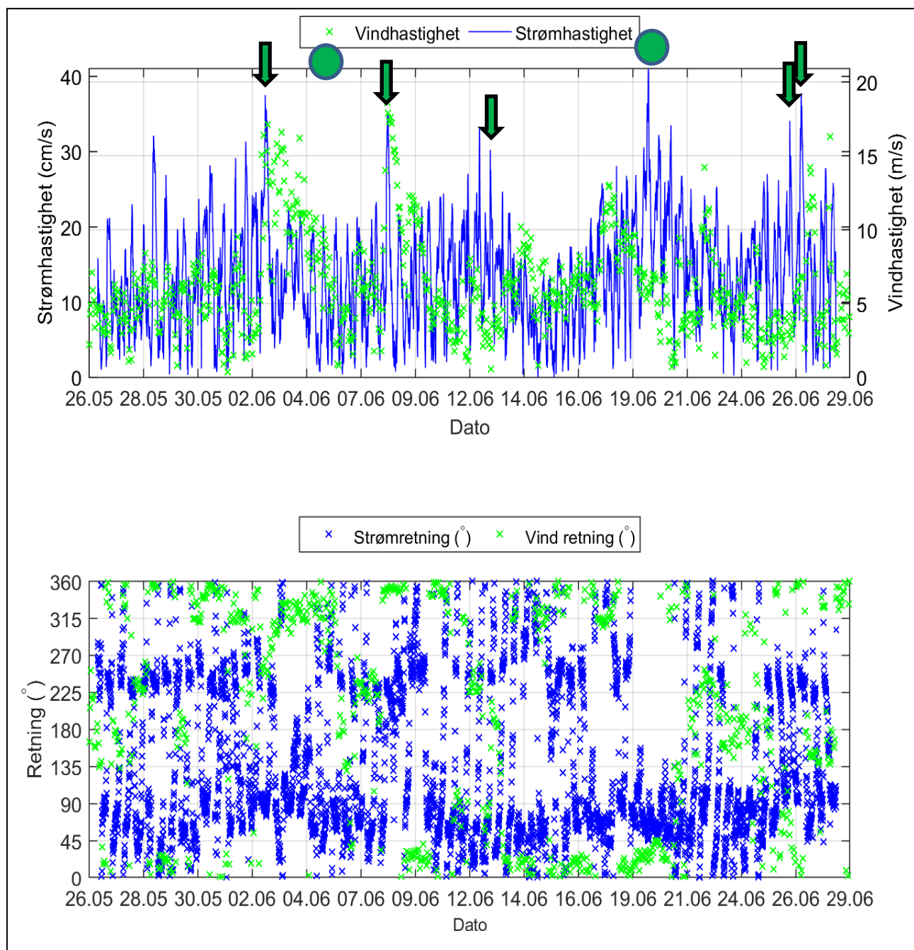
Figur 4.22.2. Strømhastighet på 5m og vindhastighet og strøm og vind retning (Fakken værstasjon) under måleperioden.
