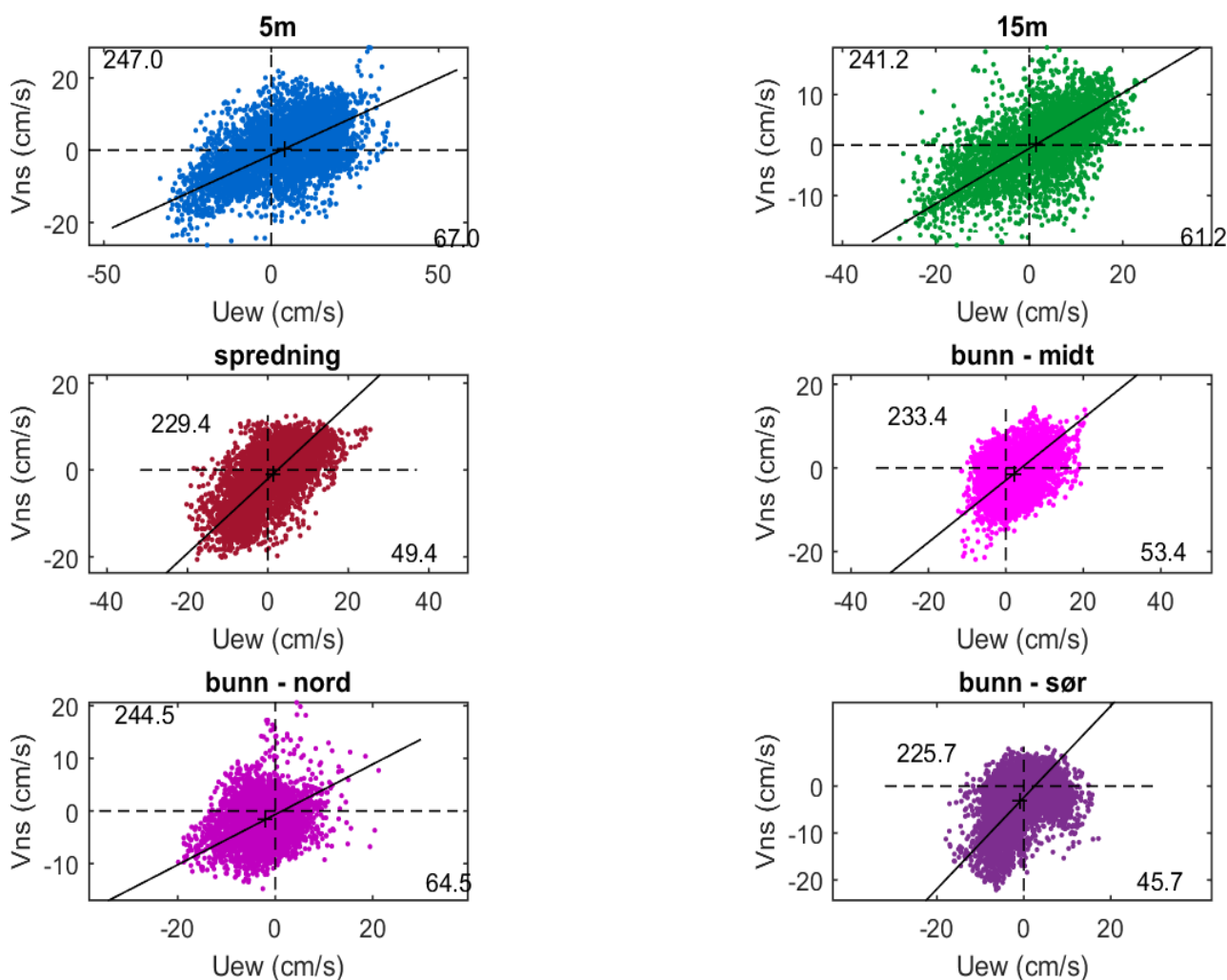
Figur 4.21.1. U_{EW} - V_{NS} punktdiagram.
