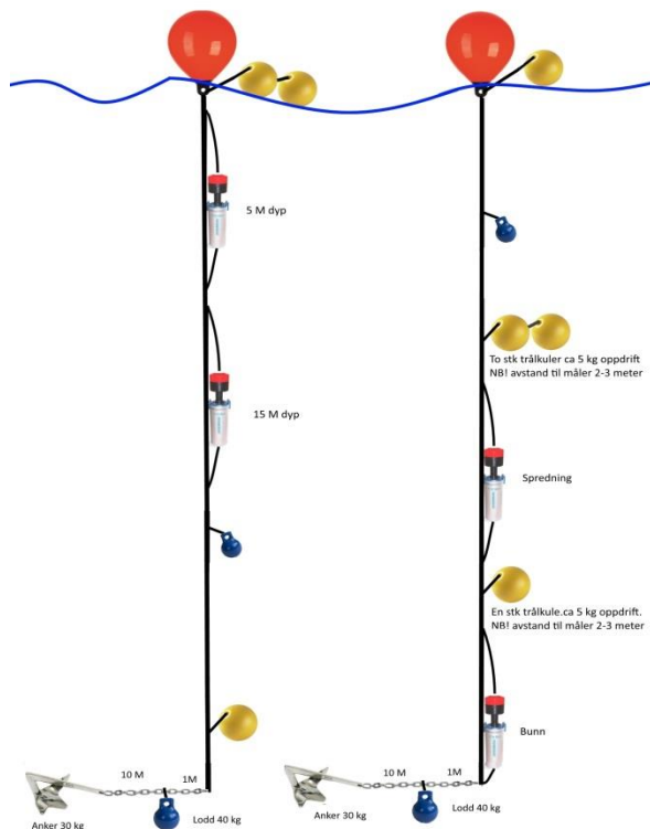
Figur 7.1.1. Skisse riggoppsett – Aanderaa punkt måler.
