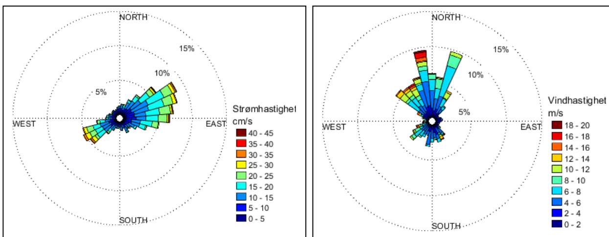
Figur 4.22.1. Rosediagram av strøm (mot retning) på 5m (venstre) og vind (fra retning) på Fakken (høyre) under måleperioden.
